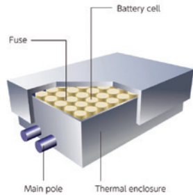
Battery Module
