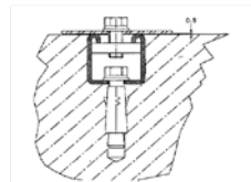
Fissaggio con ferri
