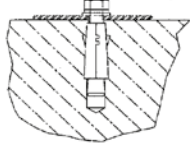
Fissaggio con viti a pavimento
