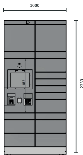
S-Box
