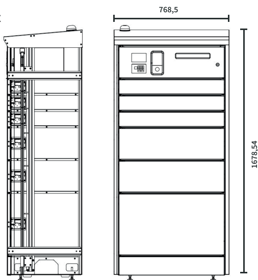
P-Box
