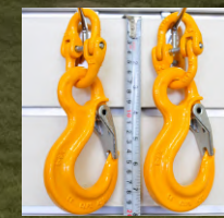
Hammerlock + Slip Hook 7/8mm*Breaking 8000kg
