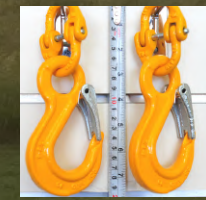
Hammerlock + Sling Hook 7/8mm*Breaking 8000kg
