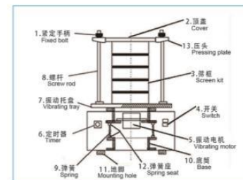
TS-200标准试验筛 TS-200 Standard test sieve
