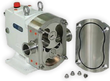
Lobe Pump مضخة اللوب
