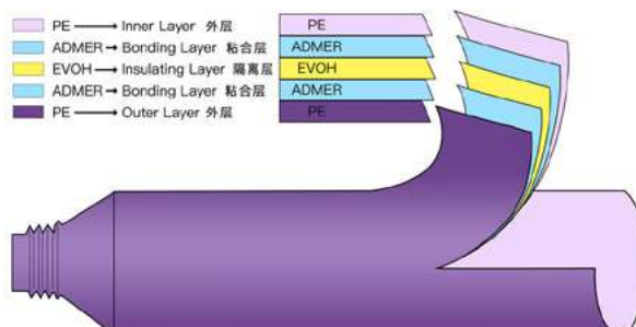
b. Five-layer PE tube 5层PE管
