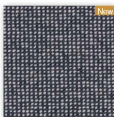
Aquarius
