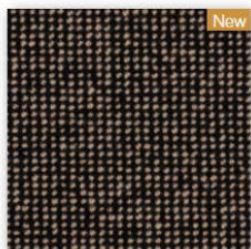
Gemini
