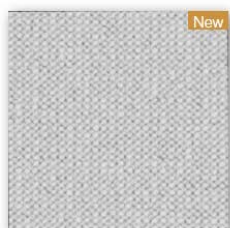
Cygnus
