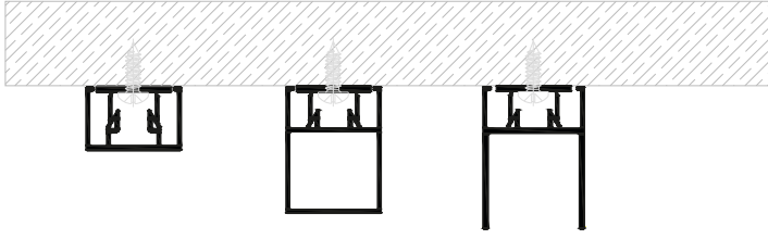
SVC04: tekil olarak kapak profilleri ile kullanılabilen versiyon SVC04: the version that can be used individually with cover profiles
