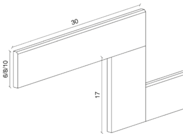
Rampante / Zoccolino a nastro Step's skirting
