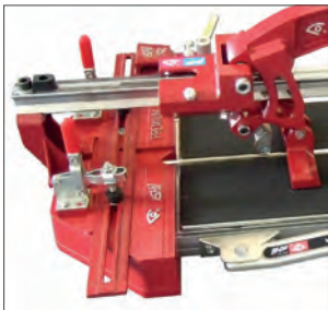
Flip-up guide
