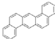
Dibenzo(a,h)anthracene
